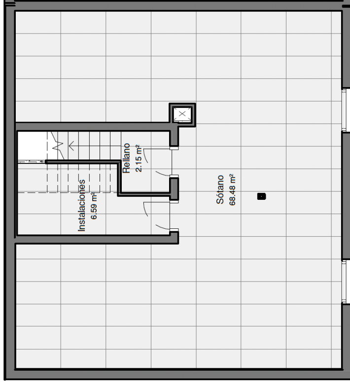
PLANTA SÓTANO
